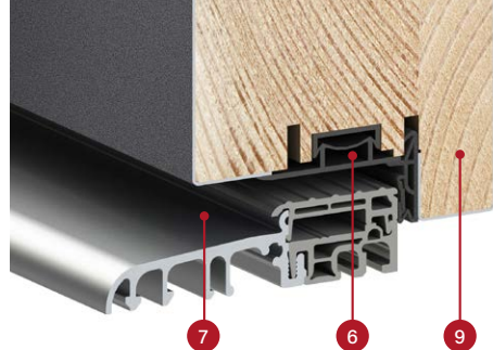
prerez krila THERMO HOT 78 s tesnilom in brez avtomatskega tesnila, alu prag
