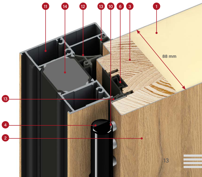
prerez alu podboja za krilo THERMO HOT 88
