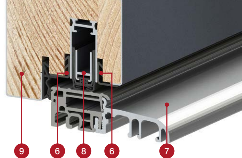
prerez krila THERMO 64 s tesnilom in brez avtomatskega tesnila, alu prag
